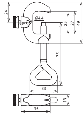
Maßbild PK 2.21 ASSM5 TGTZN
