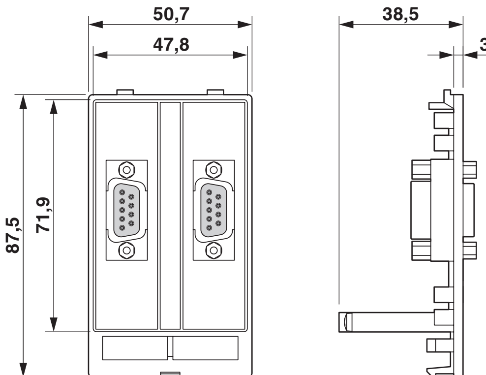
Dessin coté
