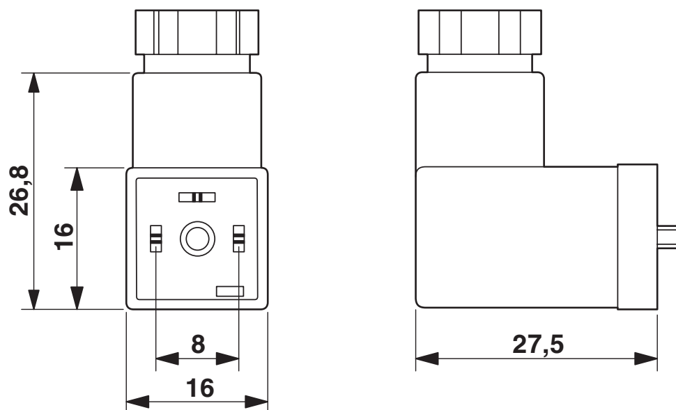
Dessin coté
