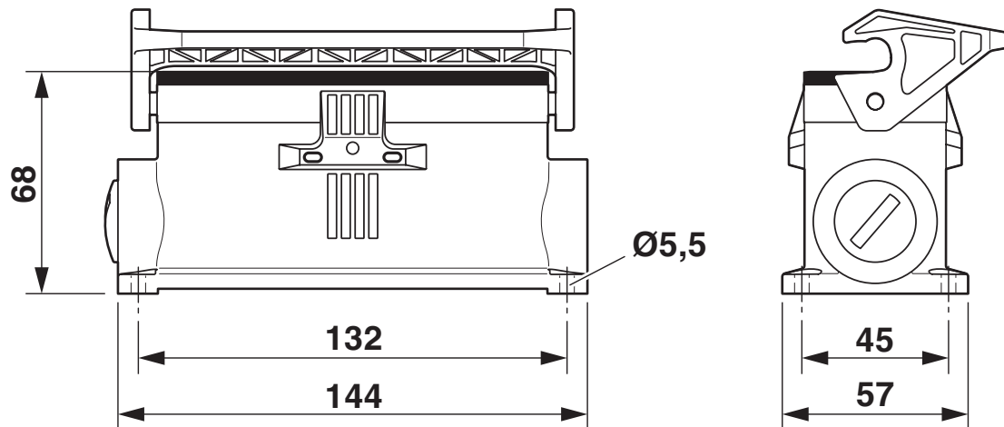
Maßzeichnung
