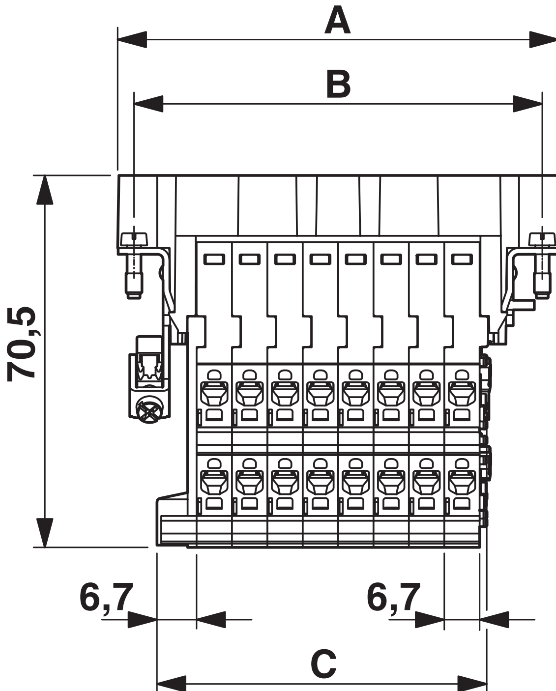
Maßzeichnung
