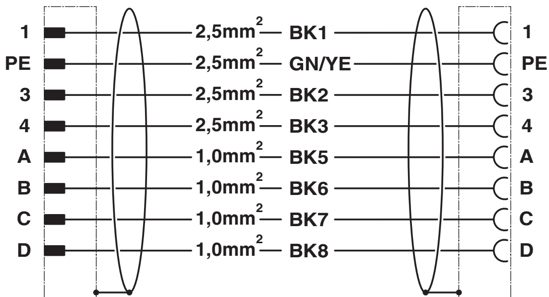
Diagrama eléctrico
