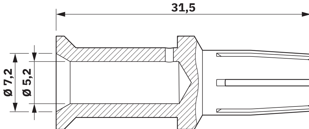
Maßzeichnung
