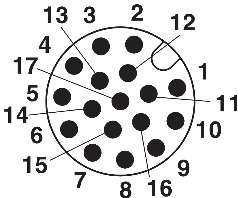
Dessin schématique
