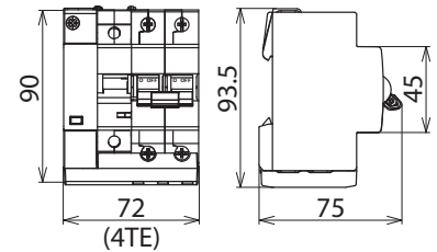
Maßbild SPD+POP 2 255 C40
