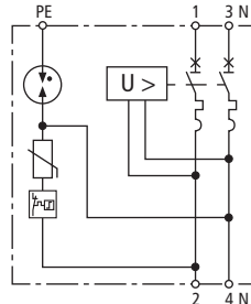
Prinzipialschaltbild SPD+POP 2 255 C40
