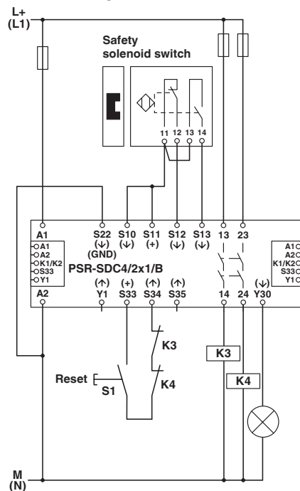
Diagrama eléctrico
