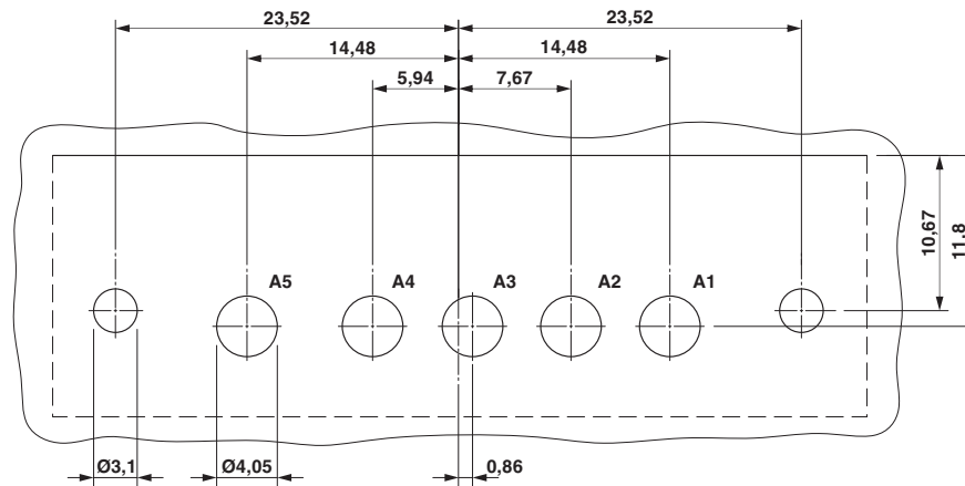
Bohrplan/Lötpadgeometrie
