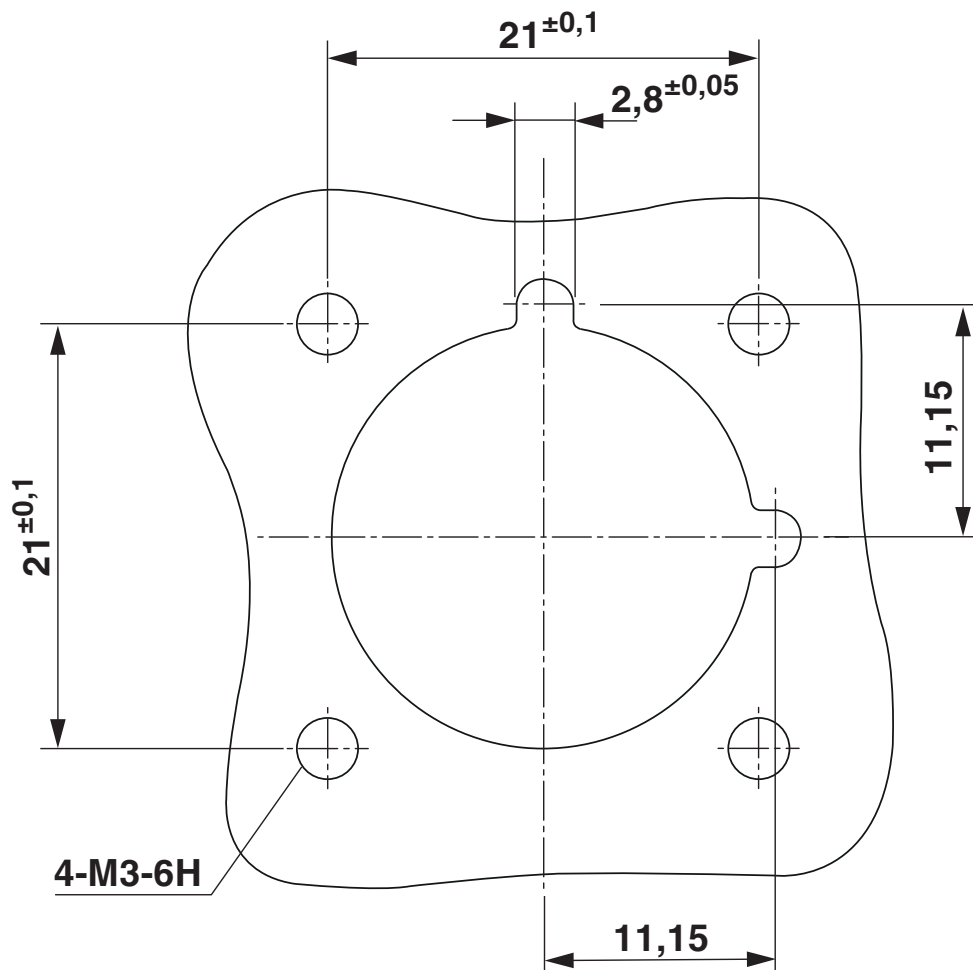
Bohrplan/Lötpadgeometrie
