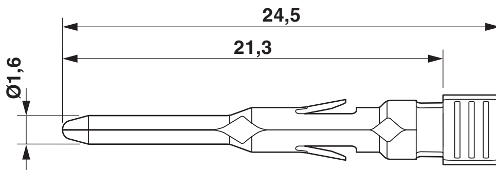
Dessin coté
