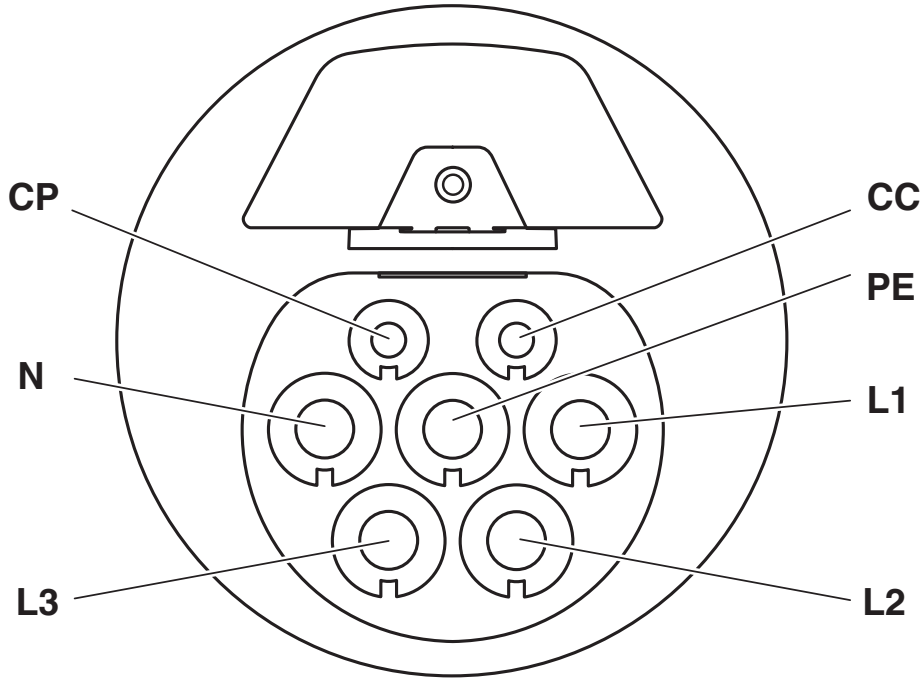
Esquema de polos de entradas de carga para vehículos
