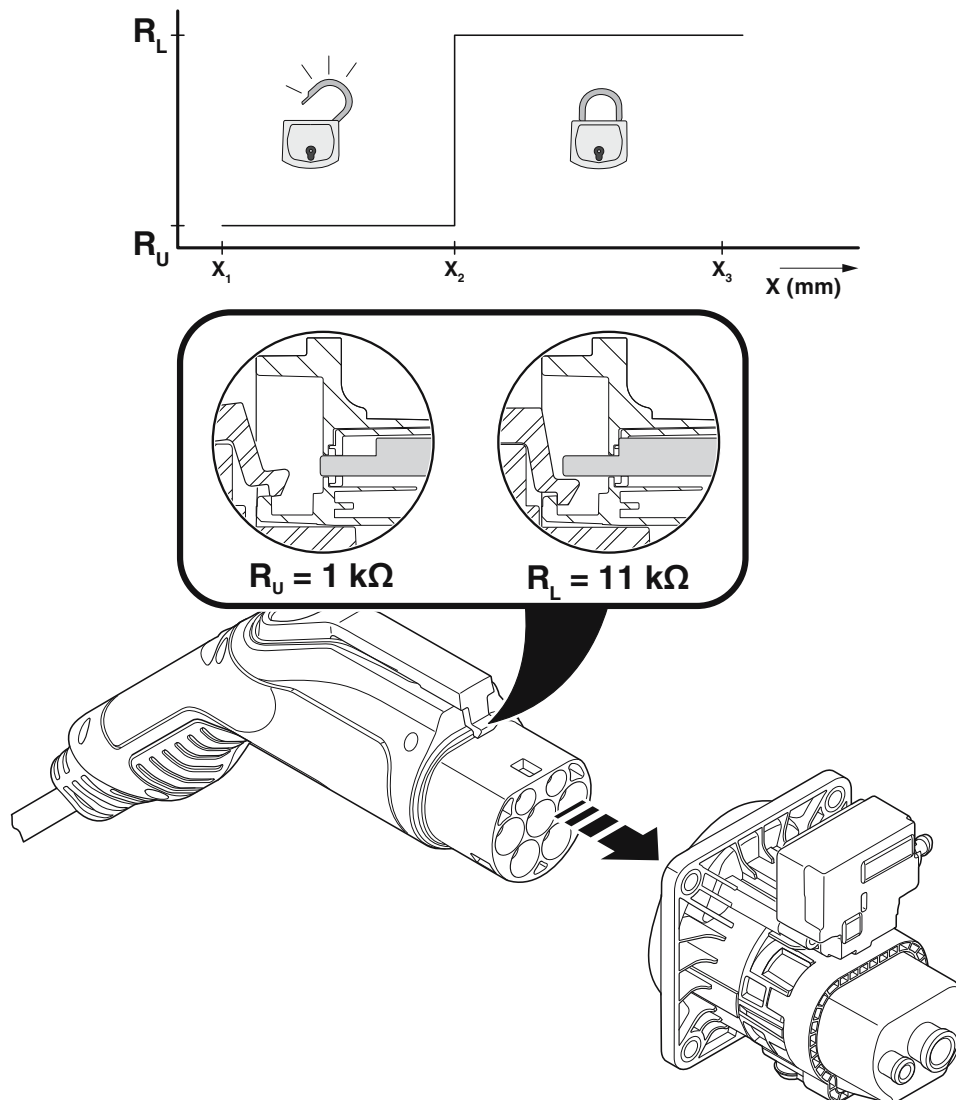
Plano esquemático
