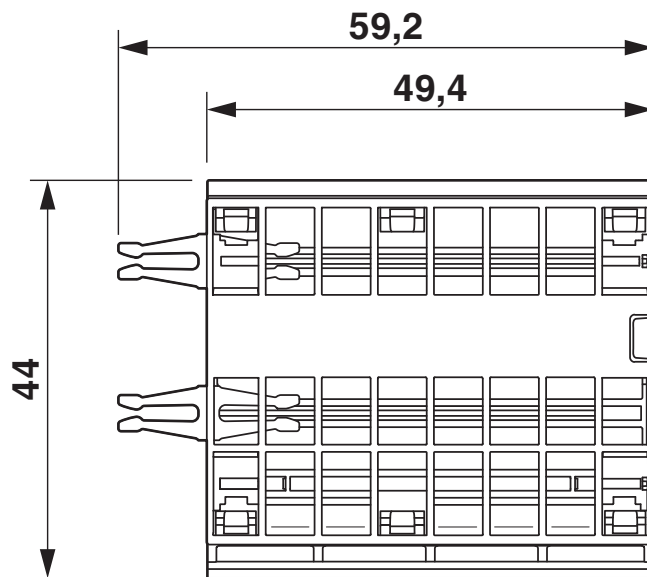
Dessin coté
