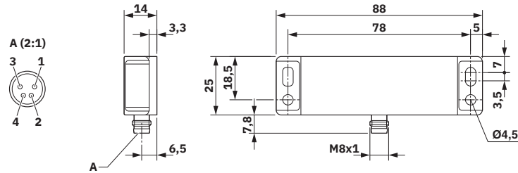
Maßzeichnung
