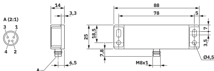
Esquema de dimensiones
