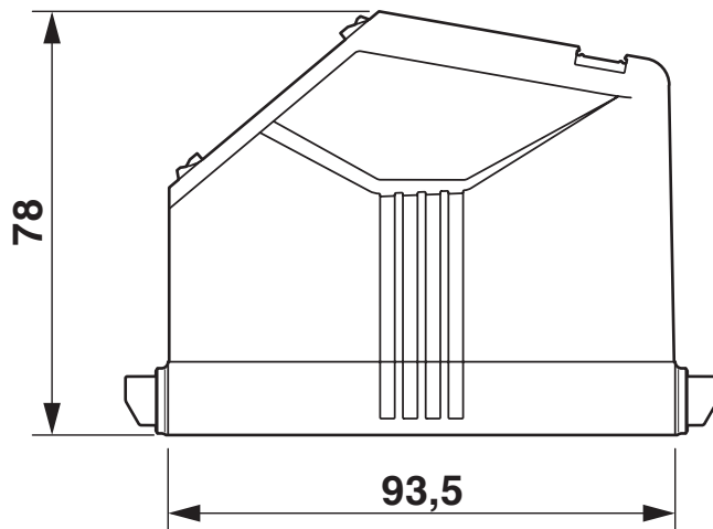
Maßzeichnung
