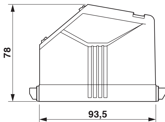
Dessin coté
