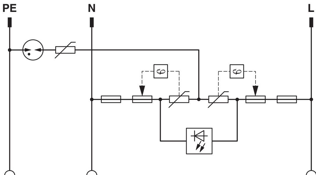
Schaltplan
