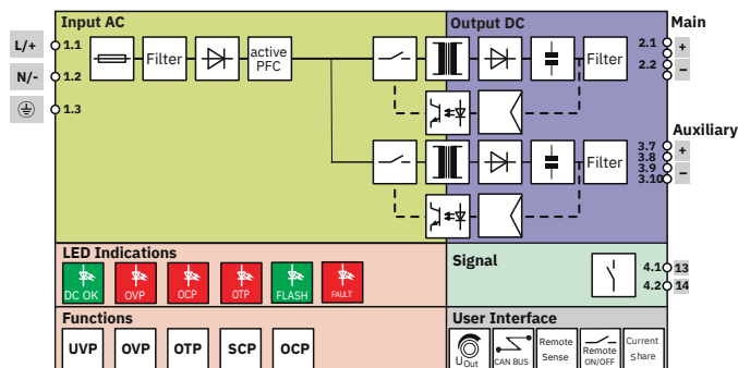
Blockschaltbild
