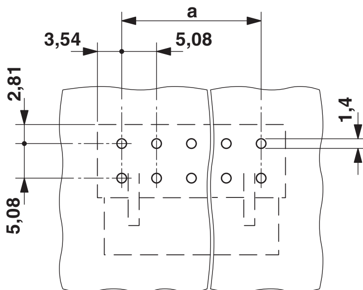
Bohrplan/Lötpadgeometrie
