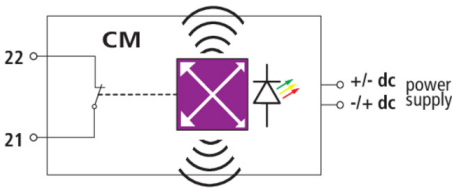
Schema di principio DRC SCM XT
