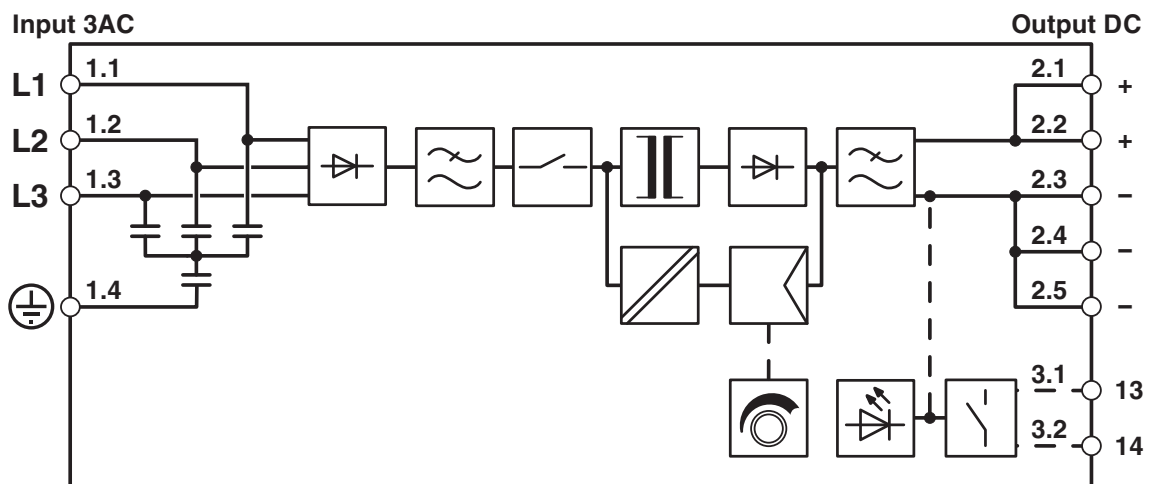
Blockschaltbild
