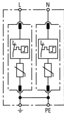
Esquema del DG M TN 275
