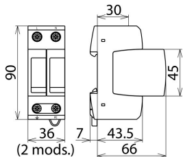
Dimesndiones del DG M TN 275
