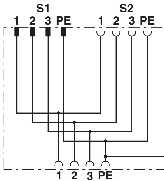
Diagrama eléctrico
