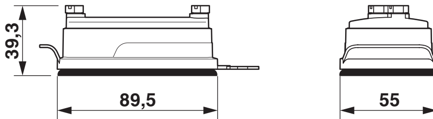
Maßzeichnung
