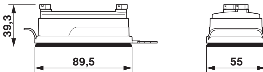
Esquema de dimensiones
