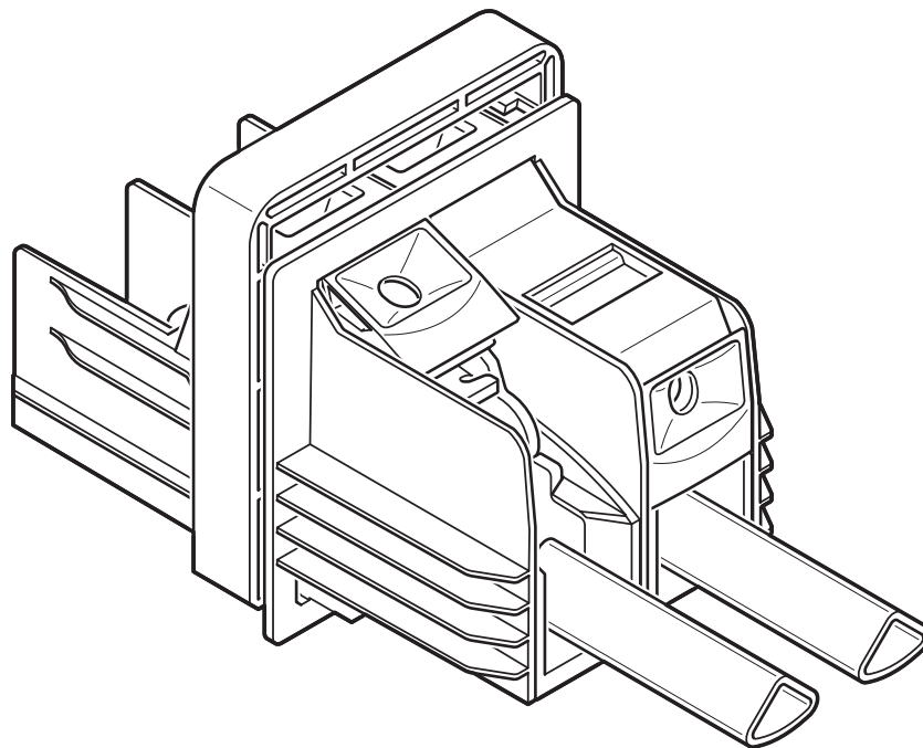
Schemazeichnung
