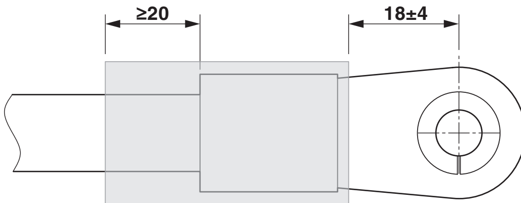
Maßzeichnung
