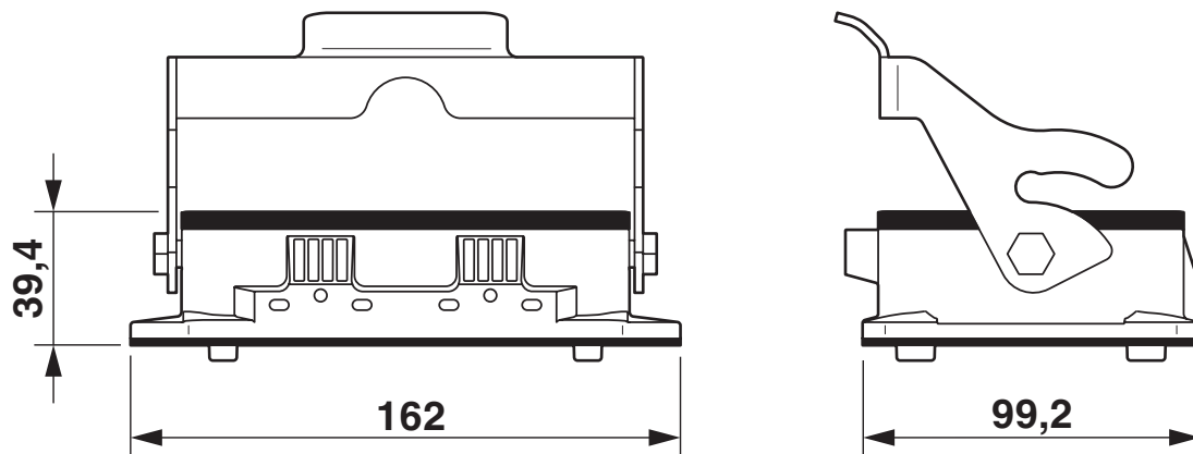
Maßzeichnung
