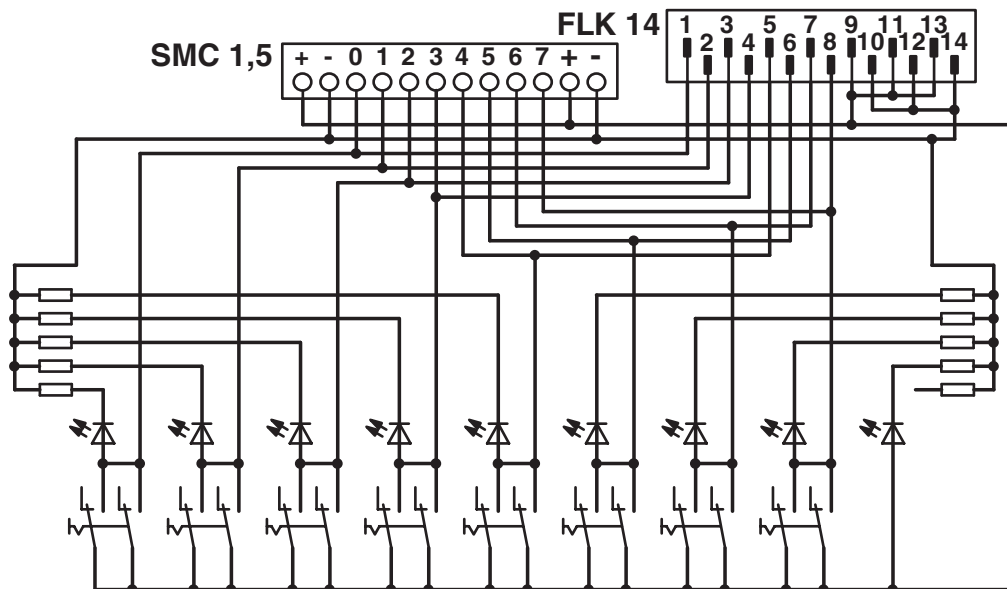
Anschlussbild UM 45-DI/DO/S/LA/SIM8
