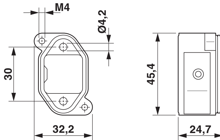
Maßzeichnung
