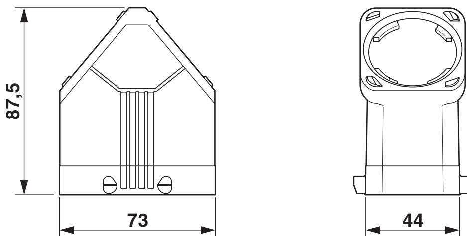
Dessin coté
