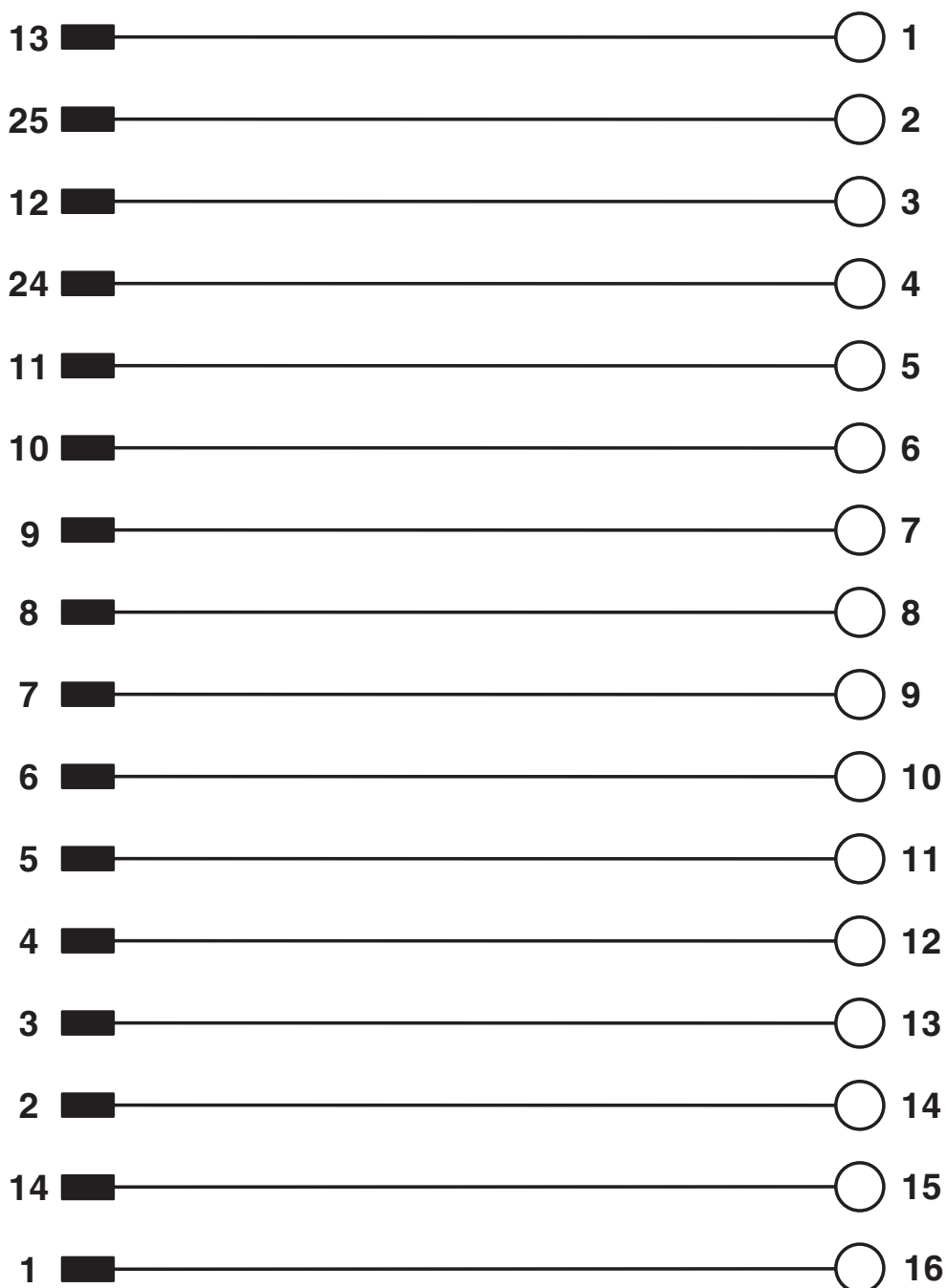
Schéma de connexion
