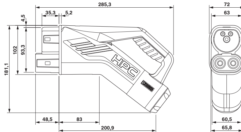
Maßzeichnung
