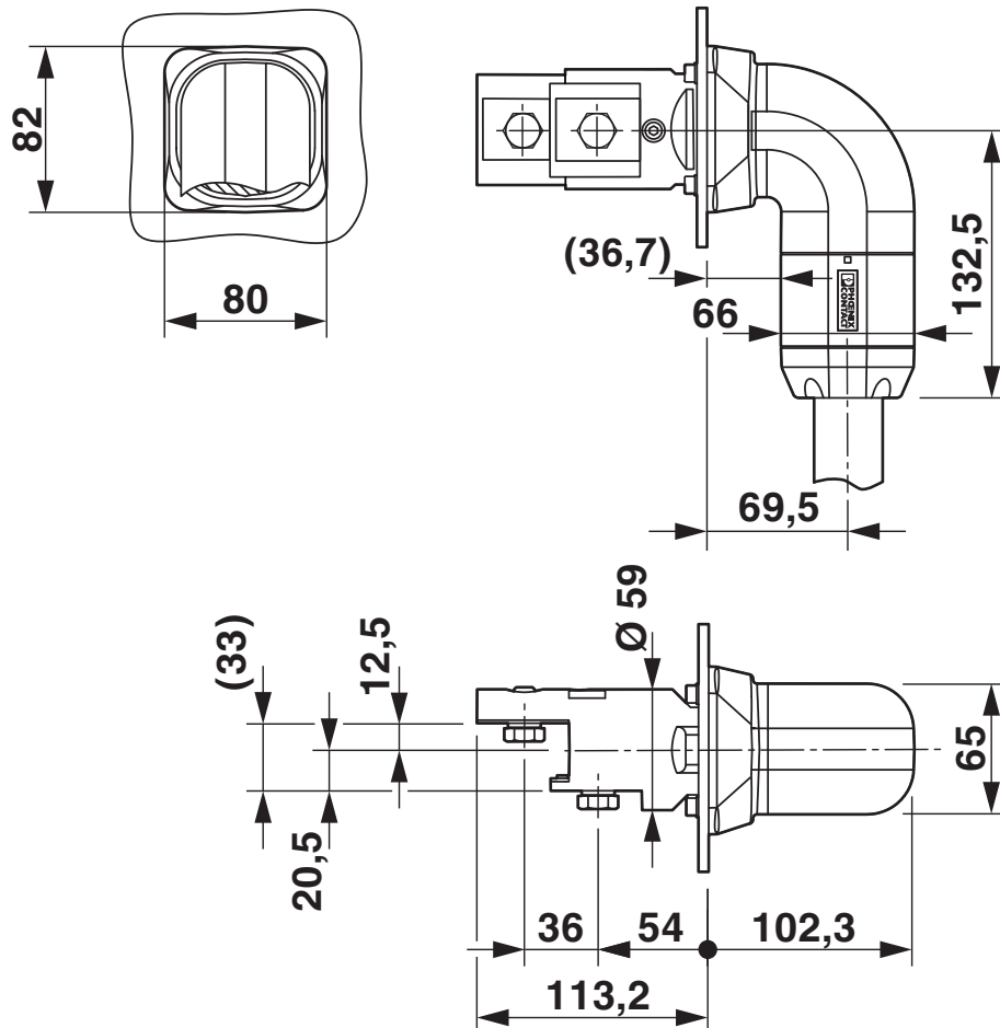
Dessin coté
