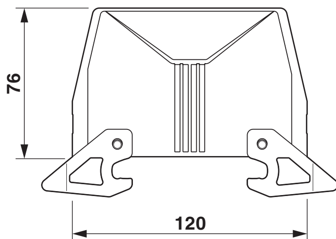
Dessin coté
