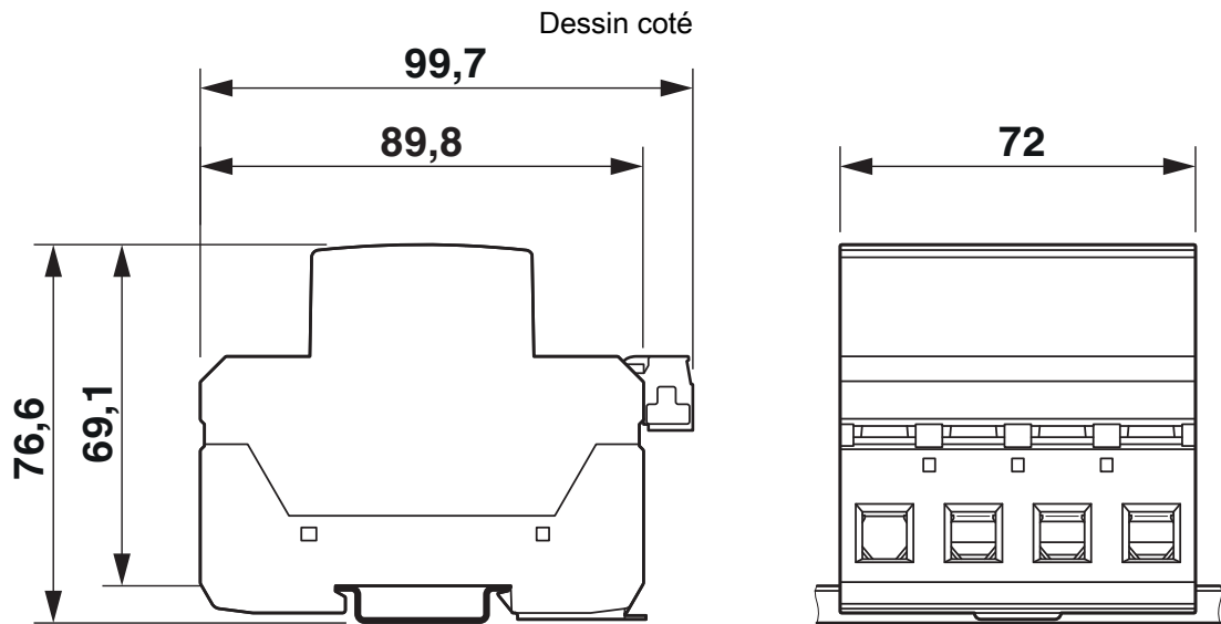
Dessin schématique
