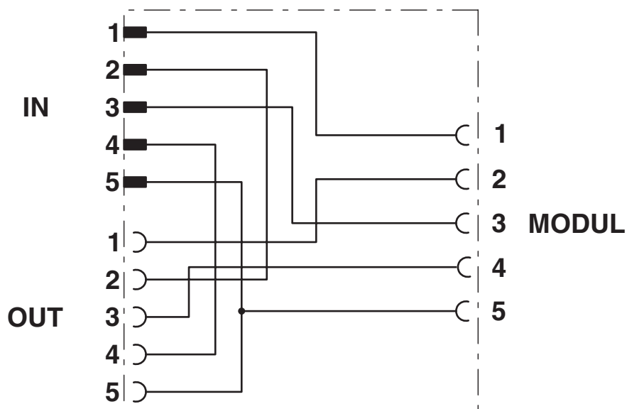
Asignación de contactos del distribuidor M12 Y
