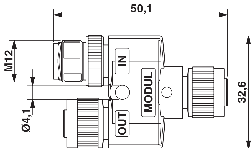
Dessin coté
