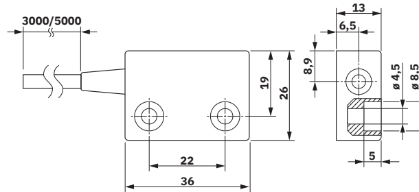
Maßzeichnung
