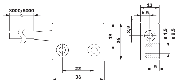
Esquema de dimensiones
