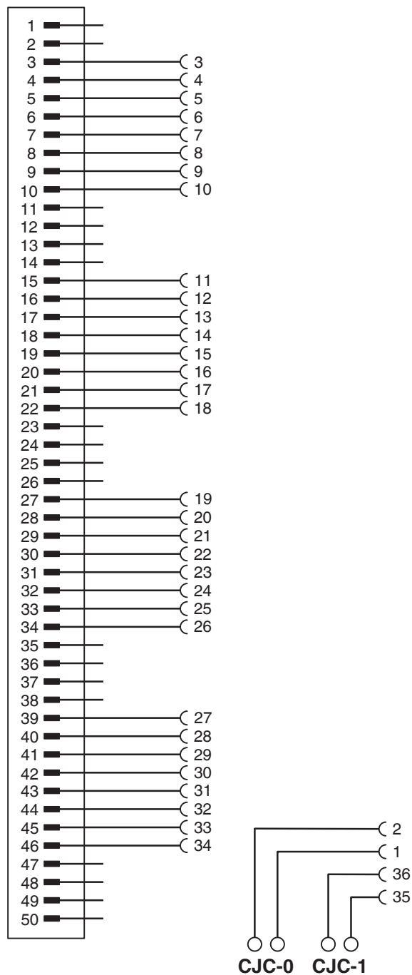
Diagrama eléctrico
