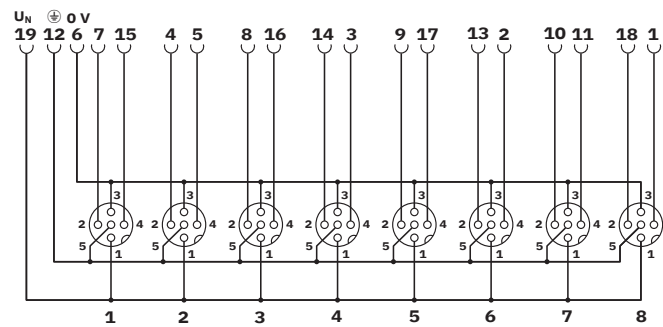
Diagrama eléctrico
