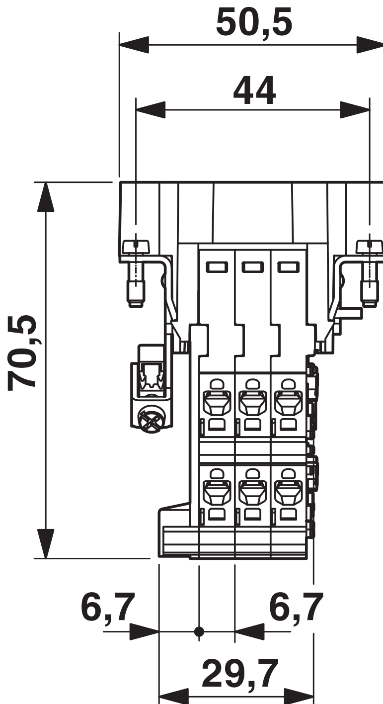
Maßzeichnung
