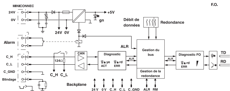
Schéma fonctionnel
