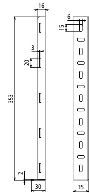
Maßbild HA SB DASD 45 D110
