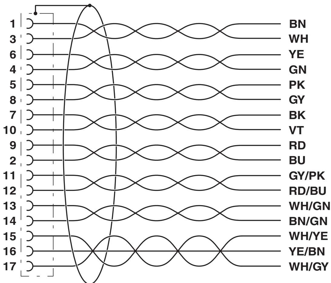
Diagrama eléctrico
