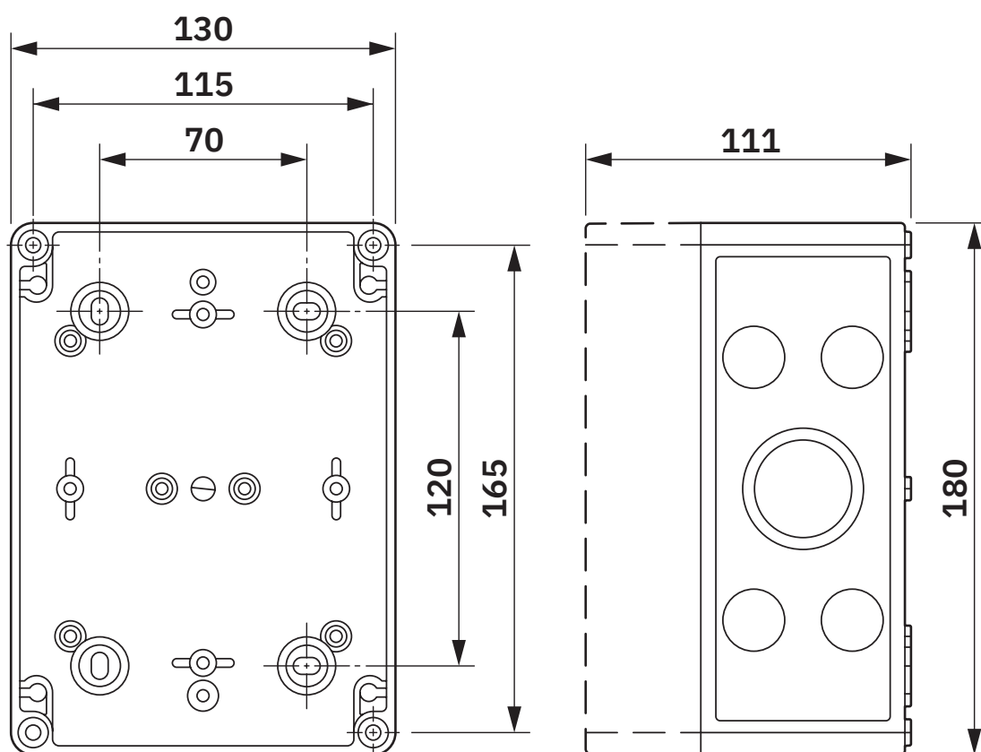
Dimensions du boîtier
