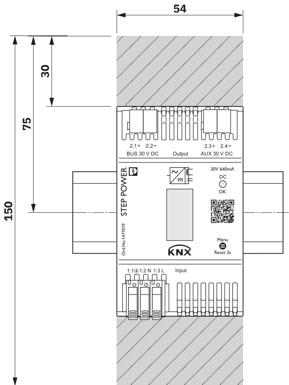
Dessin coté
